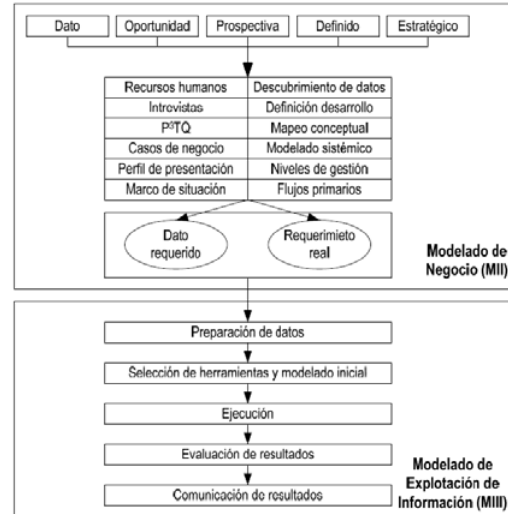
Fig. 3. Fases Metodología P3TQ
